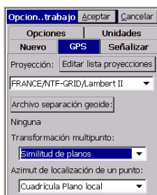
Pantalla de la ficha GPS
